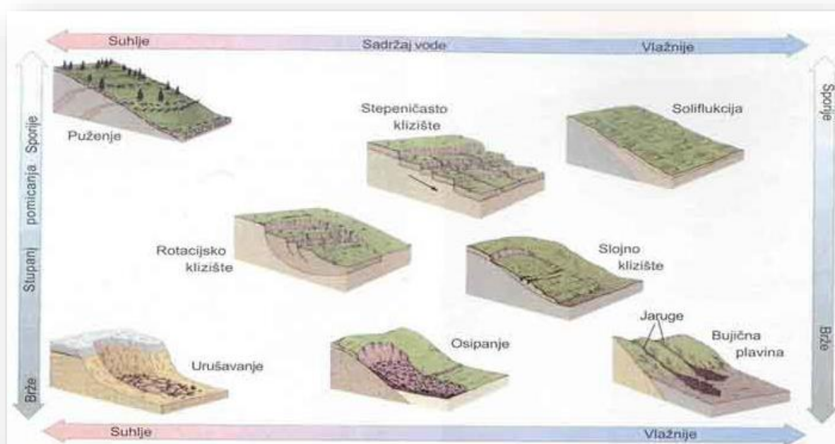
Vrste klizišta
